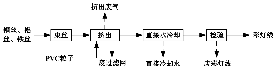
图 4-2 生产工艺及产污环节示意图
