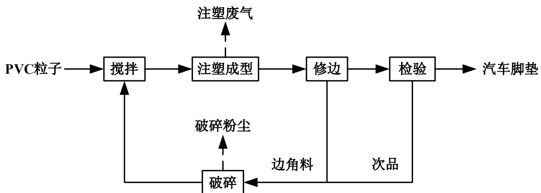
图 4-3 生产工艺及产污环节示意图
