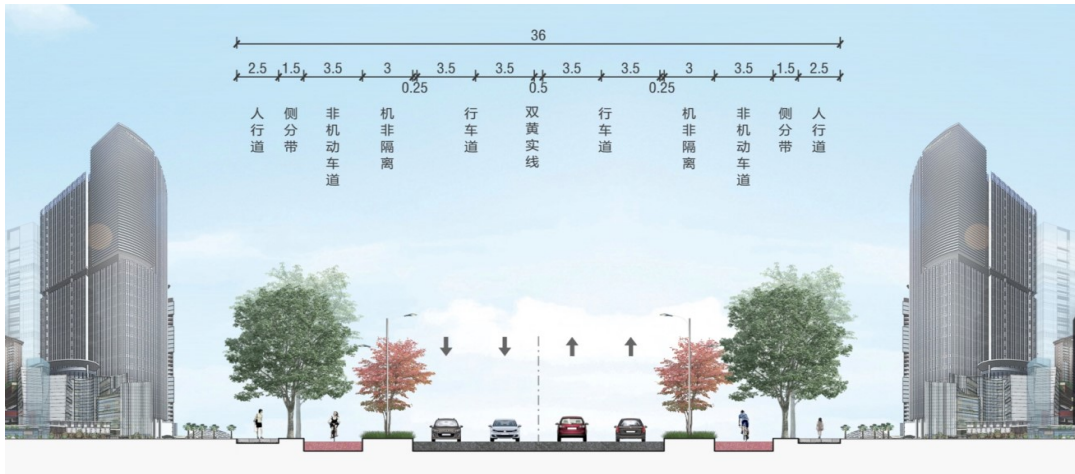
图 2-1 道路横断面布置图
