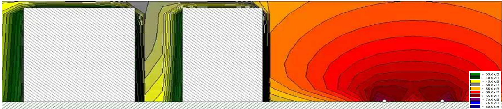
营运远期（2041 年）昼间云起玫瑰小区垂向噪声等声级线图
