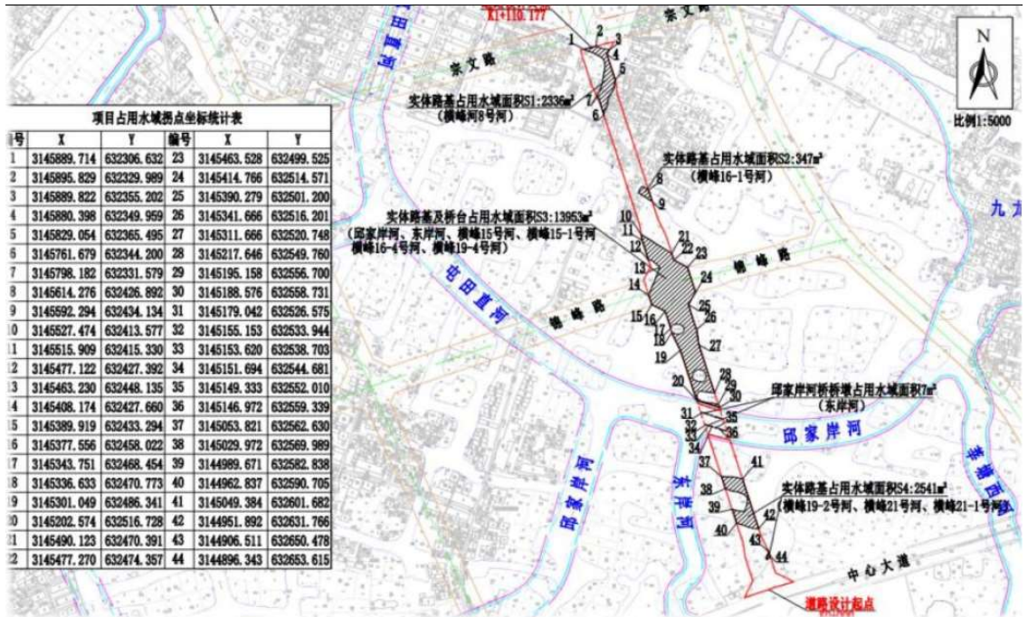
图 2-3 项目工程占用水域平面图
